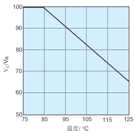
类别电压 V_C 与温度的关系
