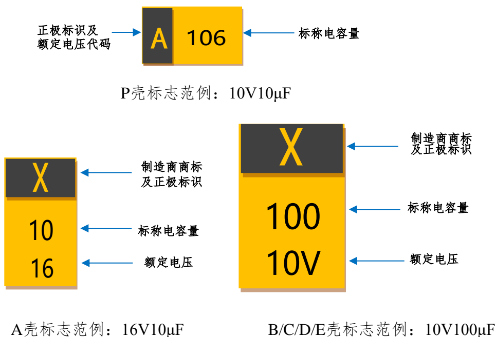
图2 钽电容器的标志示意图
