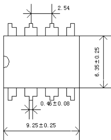
DIP8L 封装尺寸图:
