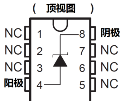
图 4 SOP8 管脚图
