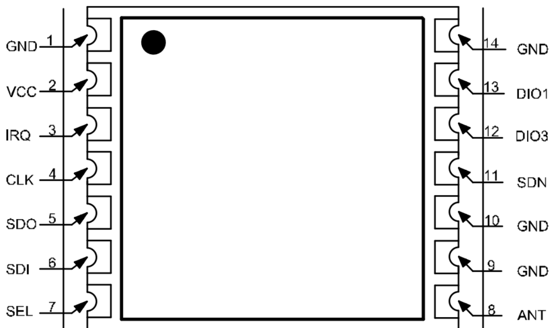
图 1-1 俯视图
