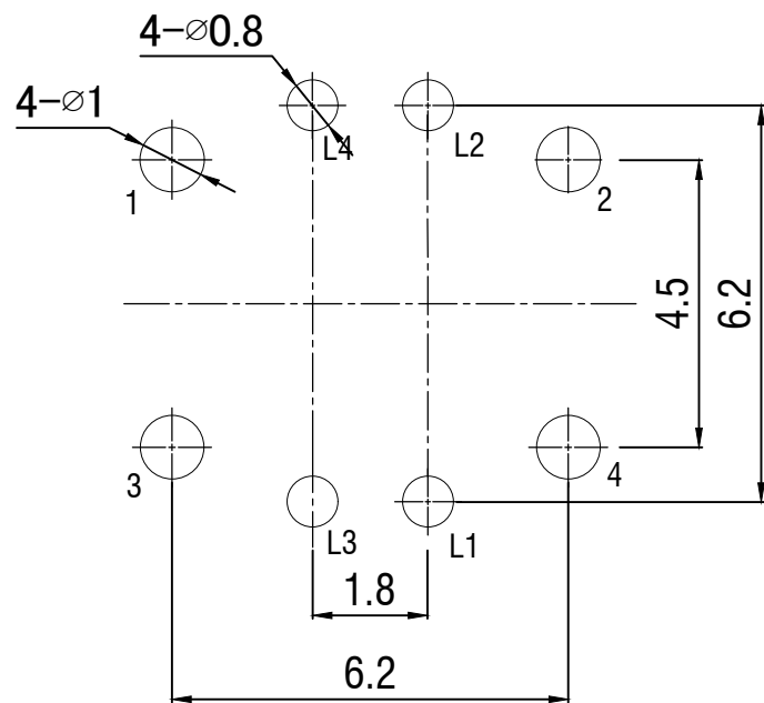
P.C.B. LAYOUT
