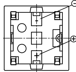
开关底部图
