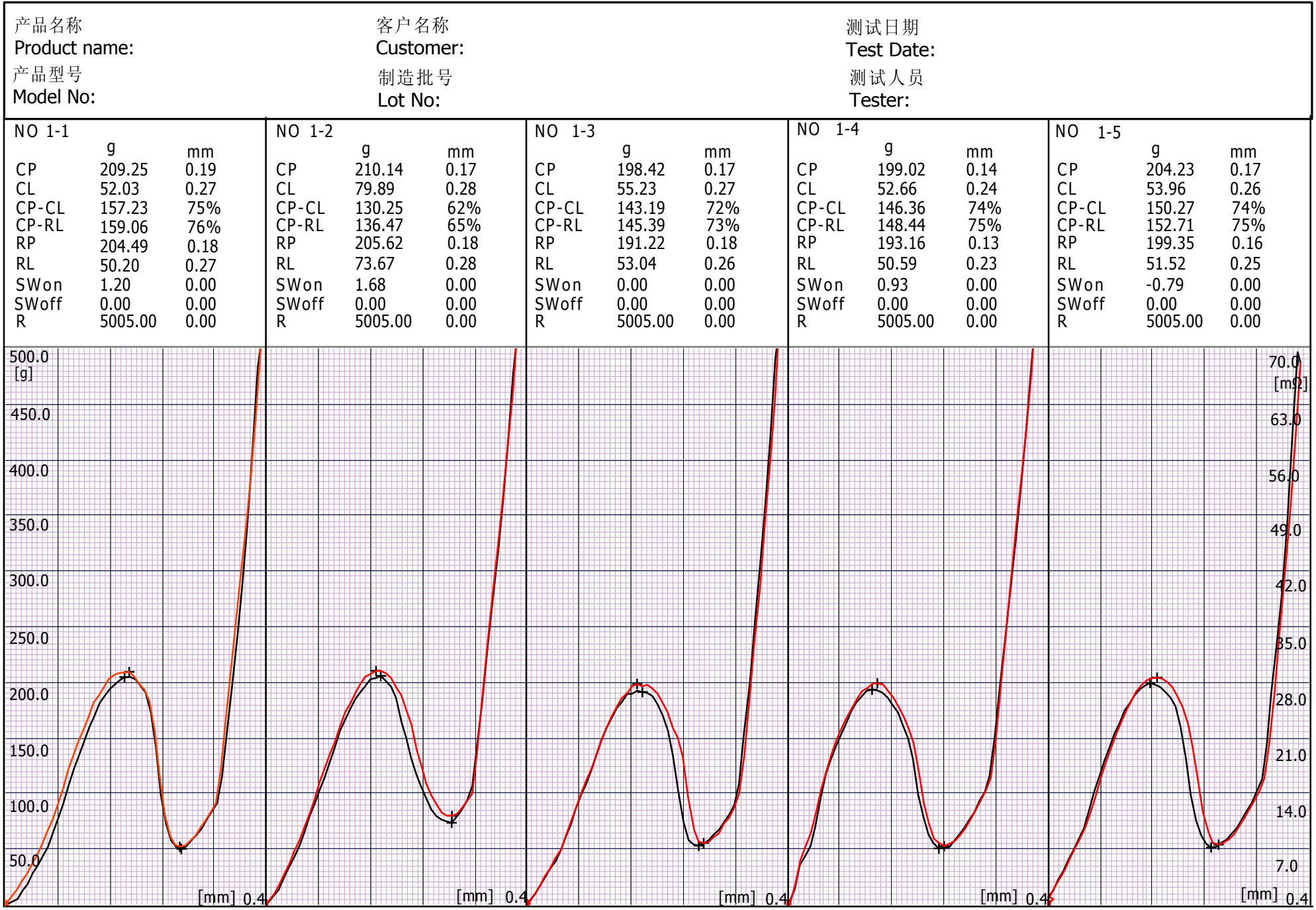
开关 (荷重-行程) 曲线
