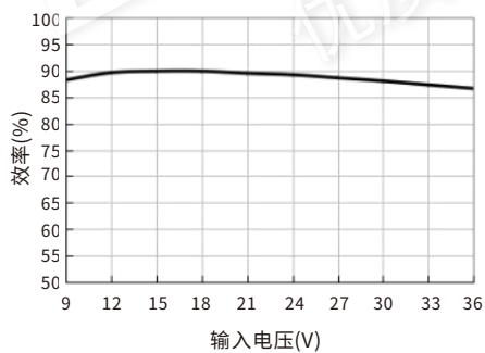
效率Vs输入电压(满载) URB2405LD-20WR3
