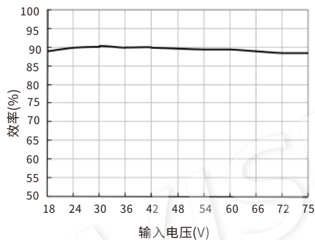
效率Vs输入电压(满载) URA4815LD-20WR3
