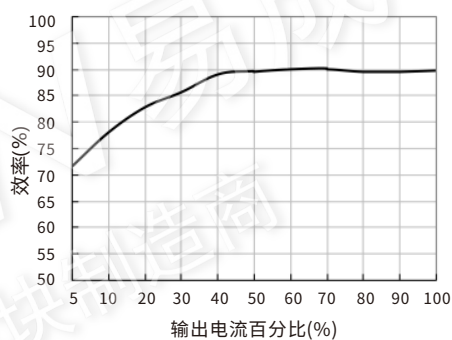
效率Vs输出负载(Vin=48V) URA4815LD-20WR3
