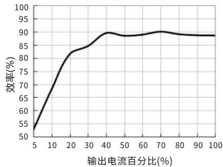
效率Vs输出负载(Vin=24V) URB2405LD-20WR3
