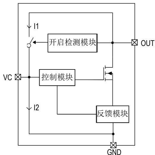
图 1. DX27641T内部功能框图
