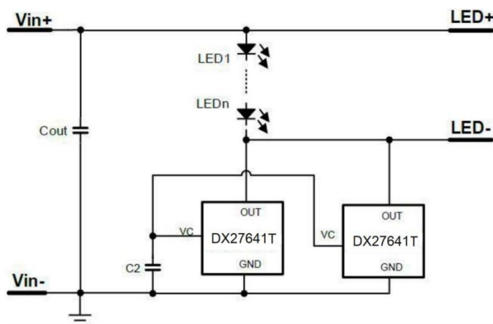
图 2. 双机并联增加输出电流
