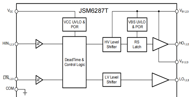
简化示意图
