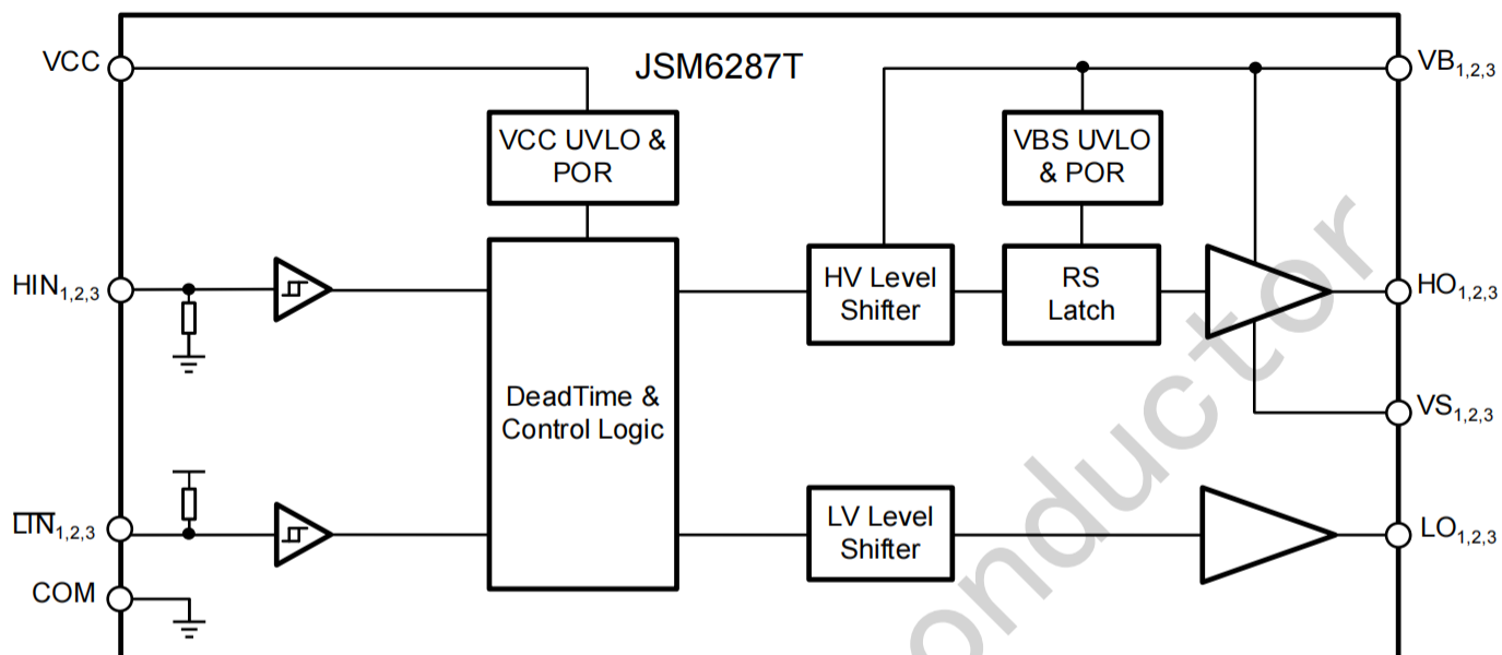
图 7-1 JSM6287T功能框图
