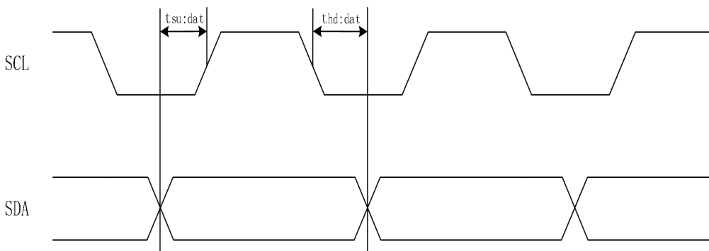
实时时钟数据传输时序
