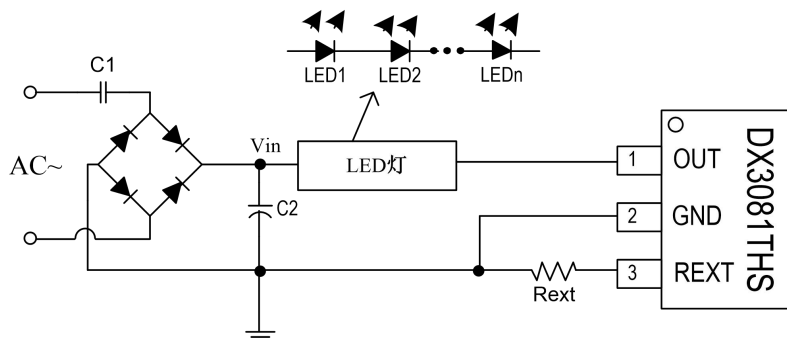
图 3. DX3081THS 典型应用电路—交流电源输入
