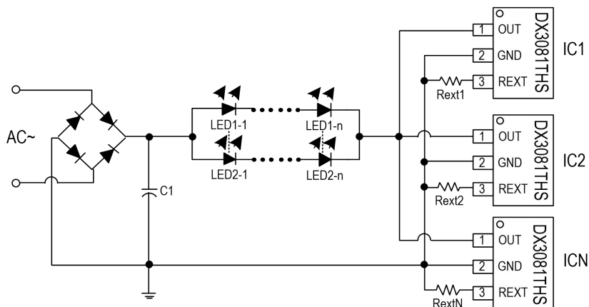
图 4. DX3081THS 并联应用电路原理图
