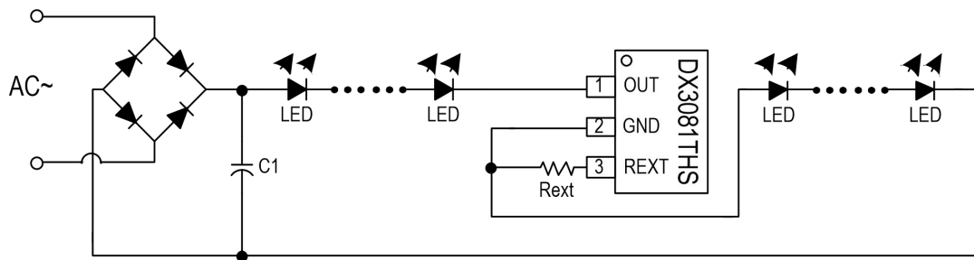
图 5. DX3081THS 串接 LED 灯管中
