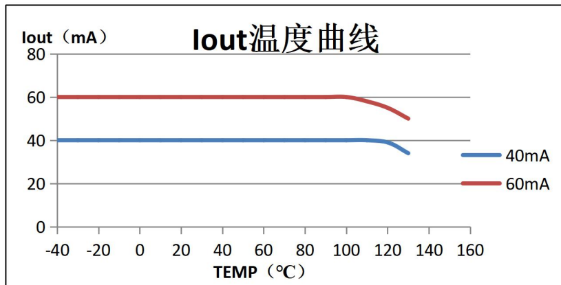
图 3. DX3081THS 输出电流温度特性
