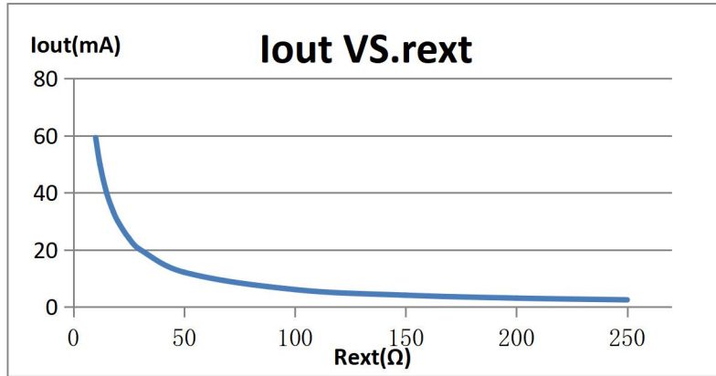
图 1. DX3081THS 输出电流与 Rext 电阻关系曲线
