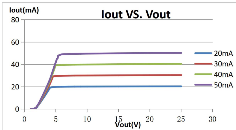
图 2. DX3081THS 恒流曲线图
