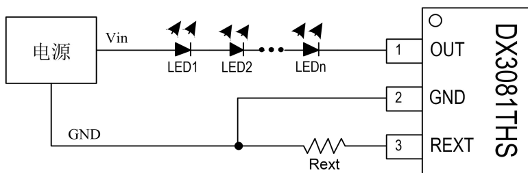
图 2. DX3081THS 应用电路原理图
