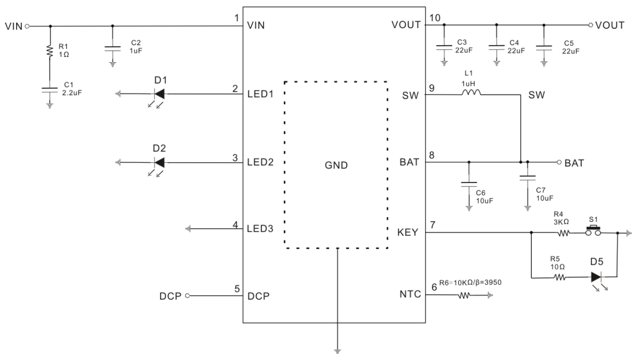
2 灯模式 (LED3 接地)
