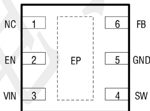
DFN-6(2X2)
