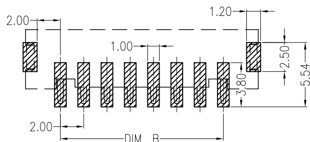
PCB Layout 线路板印刷示意图
