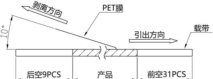
(PET膜剥离示意图)
