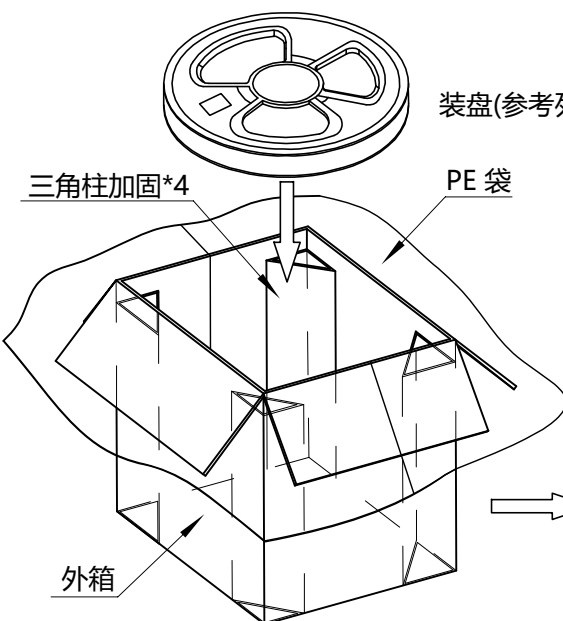
DETAIL:B
