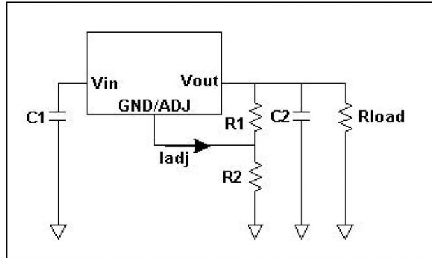
图 2 可调型应用电路
