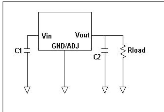
图 1 固定电压版本应用电路
