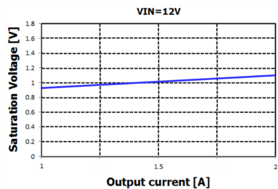
VSAT vs. IOUT
