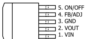
TO-263-5L
