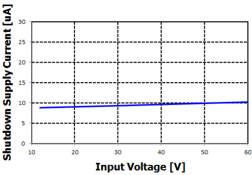
ISTB vs. VIN
