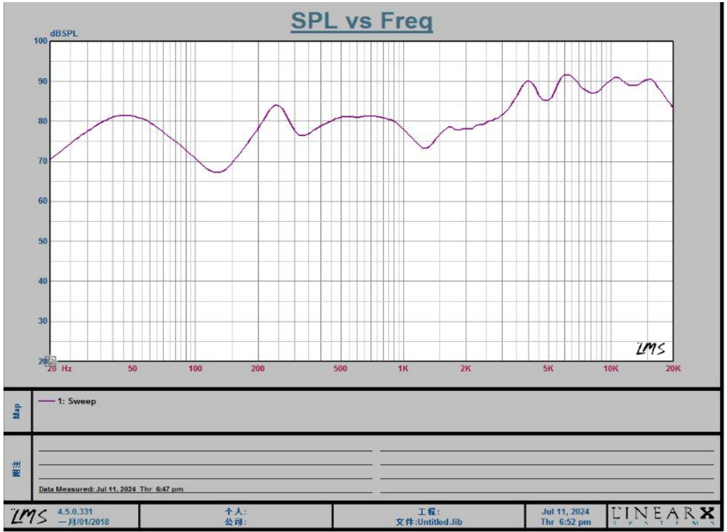
产品 SPL 曲线图 Product SPL graph
