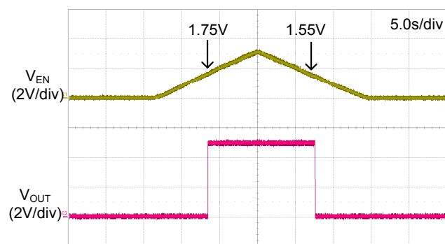
Enable Threshold
