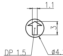
ACTUATOR
