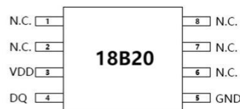
SOP8 (18B20Z)
