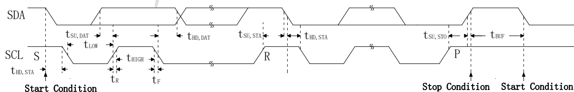
I2C 时序图
