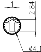
ACTUATOR
