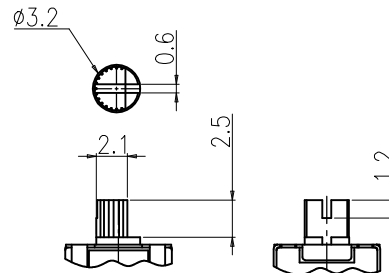
ACTUATOR
