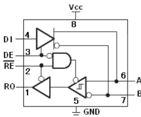
图2: JSM3085E 逻辑图
