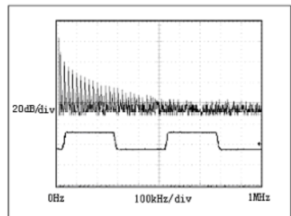
图 13: 传输 20kHz 信号时 JSM3085E驱动器输出 波形和 FFT 图
