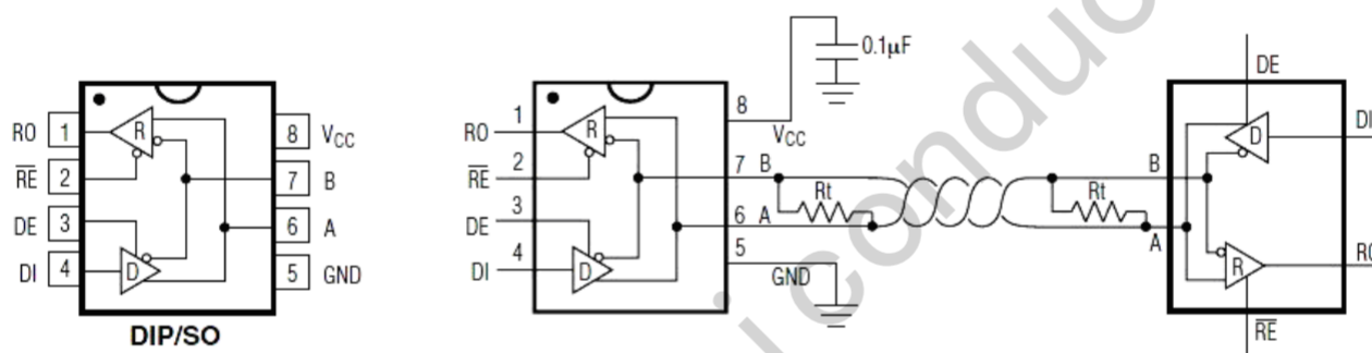
图 3: JSM3085E典型半双工应用电路
