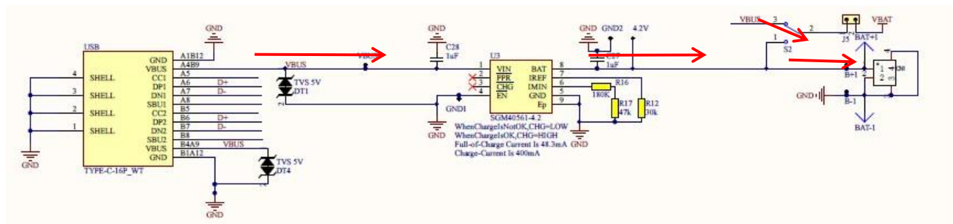
图 15 ENS001 同时对锂电池充电和为 ENS001 供电
