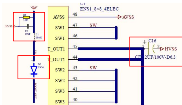
图 2 电感、电容、肖特基二极管位置
