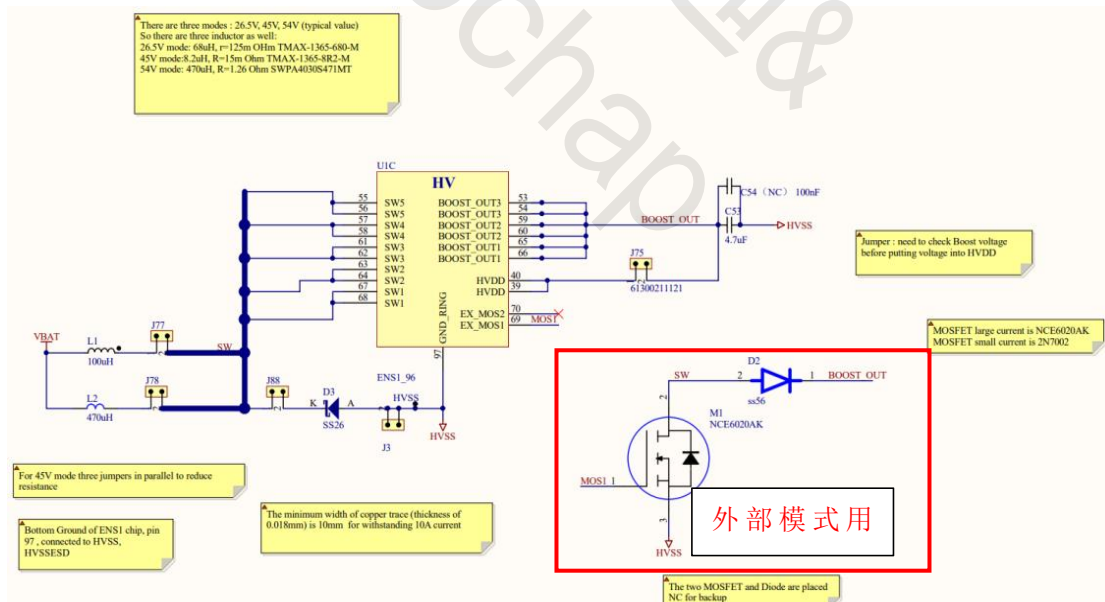
图 10 ENS001 的 BOOST 电路
