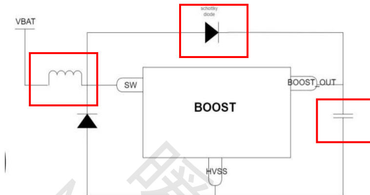
图 9 ENS001 的 BOOST 电路
