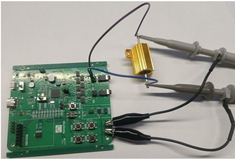
图 23 示波器探头连接方法
