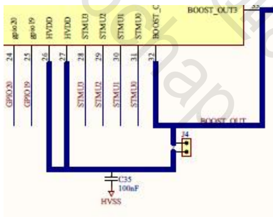
图 3 J4 跳帽原理图位置
