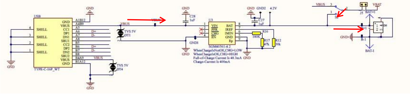
图 14 ENS001 为锂电池充电
