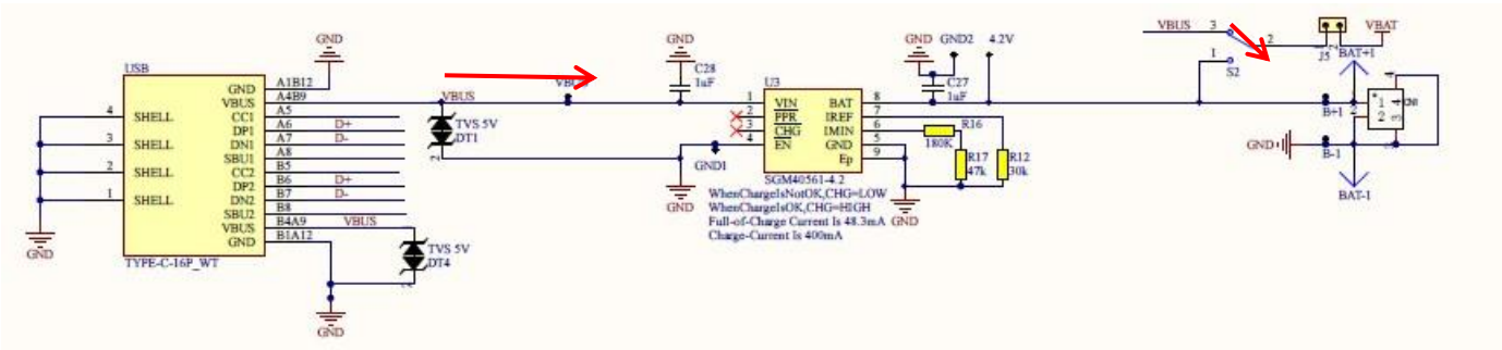
图 12 Micro USB 接口输入供电图示
