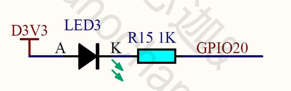
图 7 GPIO20 的 PWM 复用功能测试电路
