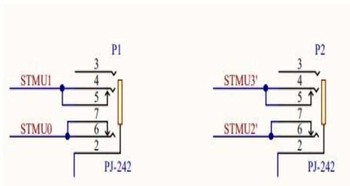
图 17 ENS001 电刺激输出耳机孔 (2 路)
