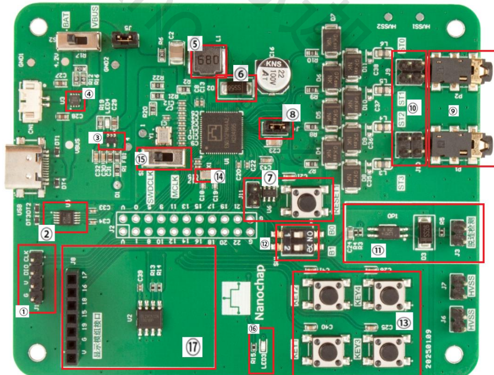
图 1 ENS1EVKE 双通道开发板图
