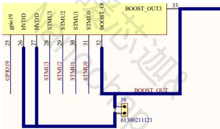
图 16 ENS001 电刺激输出引脚 STMU0~STMU3
