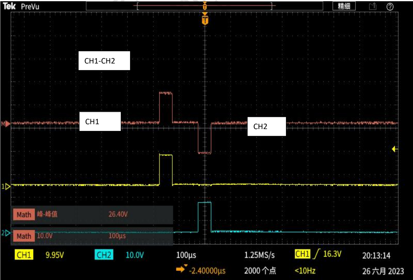
图 24 示波器处理
