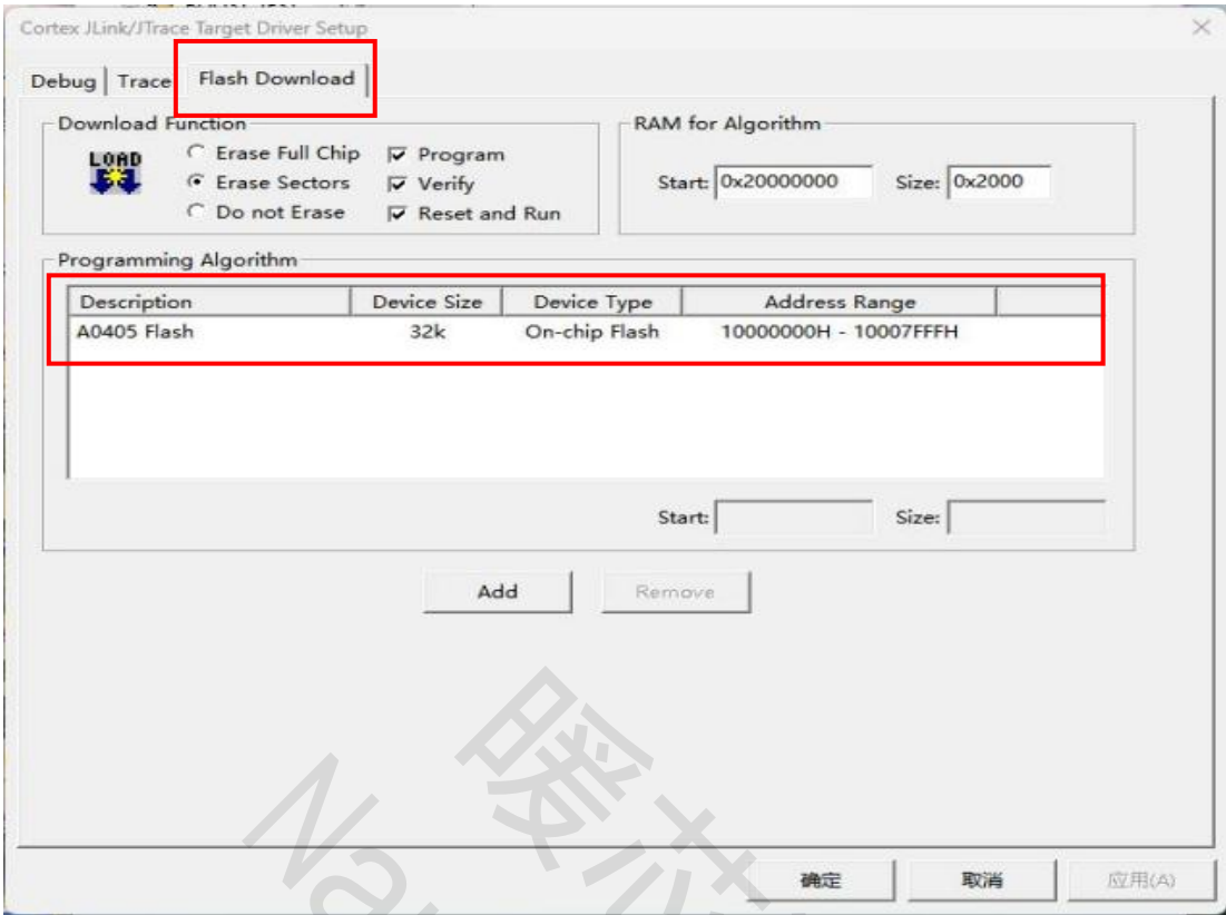
图 20 KEIL 的 flash 烧录文件选择界面
