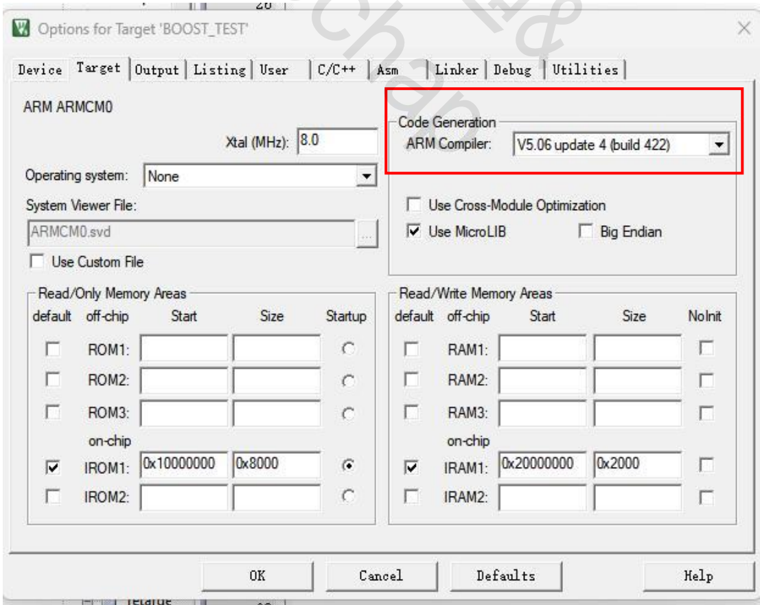
图 21 编译器选择
