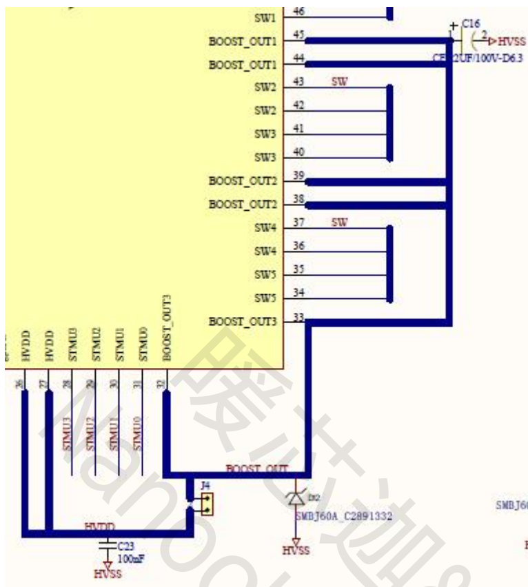
图 11 ENS001 的 boost out 和 HVDD 引脚连接
