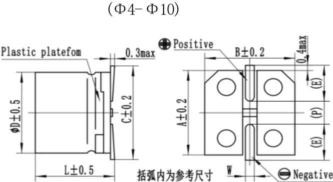
寸法图 图 1
