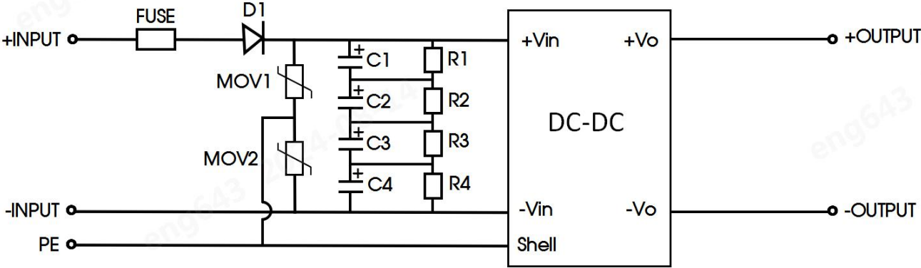
图 2: 推荐电路
