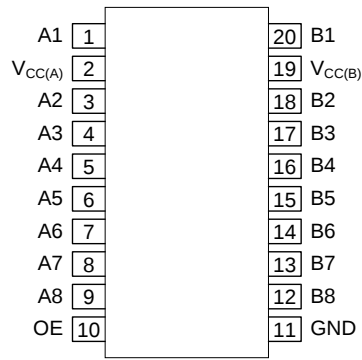
TSSOP20
