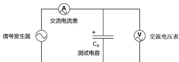
图 2 交流内阻测试电路
