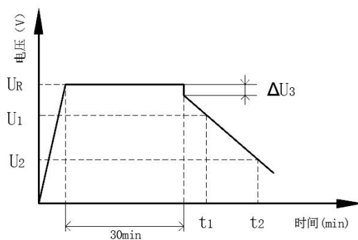
图 1 电压特性
