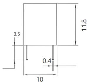
安装图
