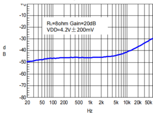
PSRR
