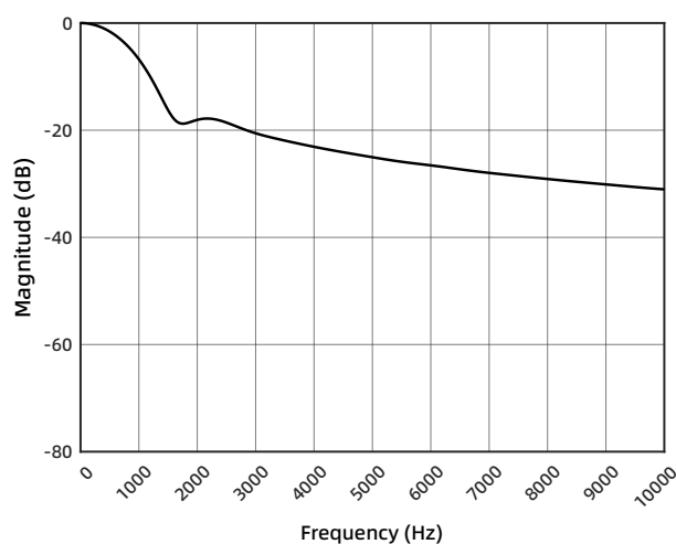
图 51 滤波器响应 (DR = 2kSPS)
