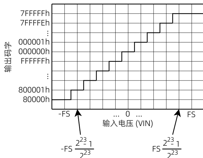
图 59 码字转换图
