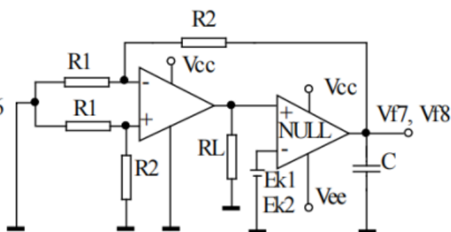
Gv = \frac{(Ek1 - Ek2)(1 + R2/R1)}{Vf8 - Vf7} 电压增益 Gv 测试图
