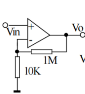
直流放大器
