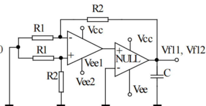
PSRR (-) = 20 \log \left| \frac{(Vee1 - Vee2)(1 + R2/R1)}{Vf11 - Vf12} \right|
