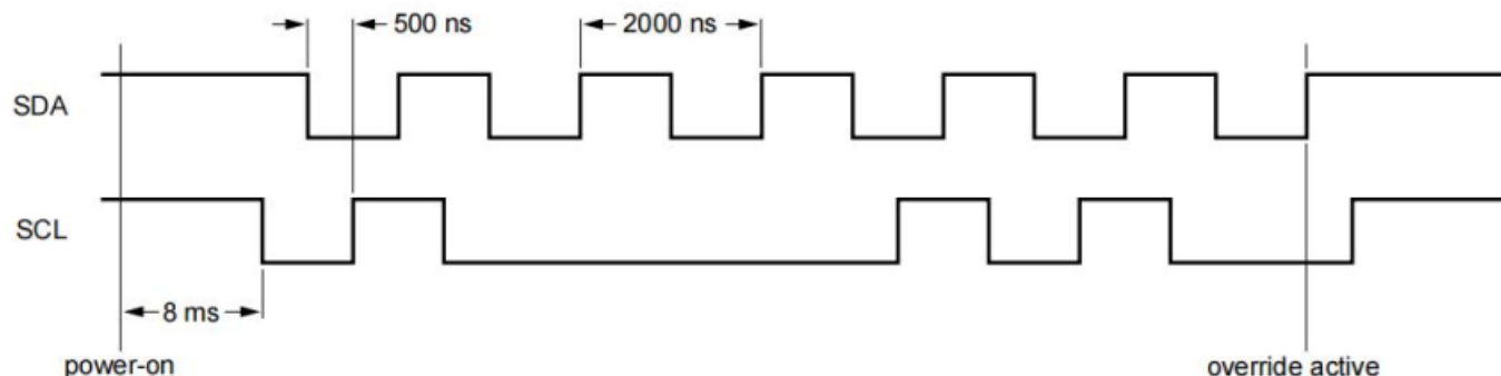
图5 POR 失败时序图
