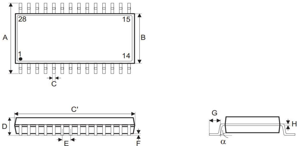
6.3 、SOP28 外形图与封装尺寸
