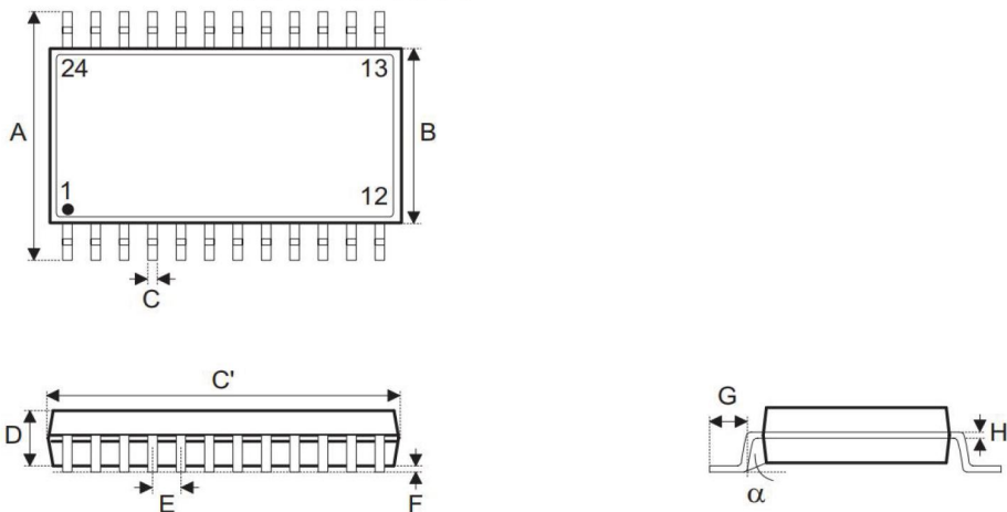
6.2、SSOP24 外形图与封装尺寸
