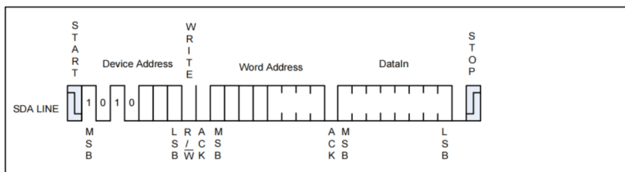
Figure5-1 ByteWrite
