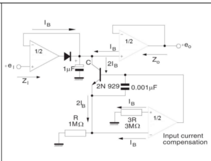
图8. 低漂移峰值检波器
