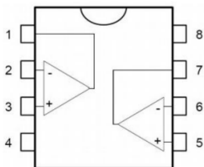
LM258(SOP8/DIP8/MSOP8/TSSOP8)
