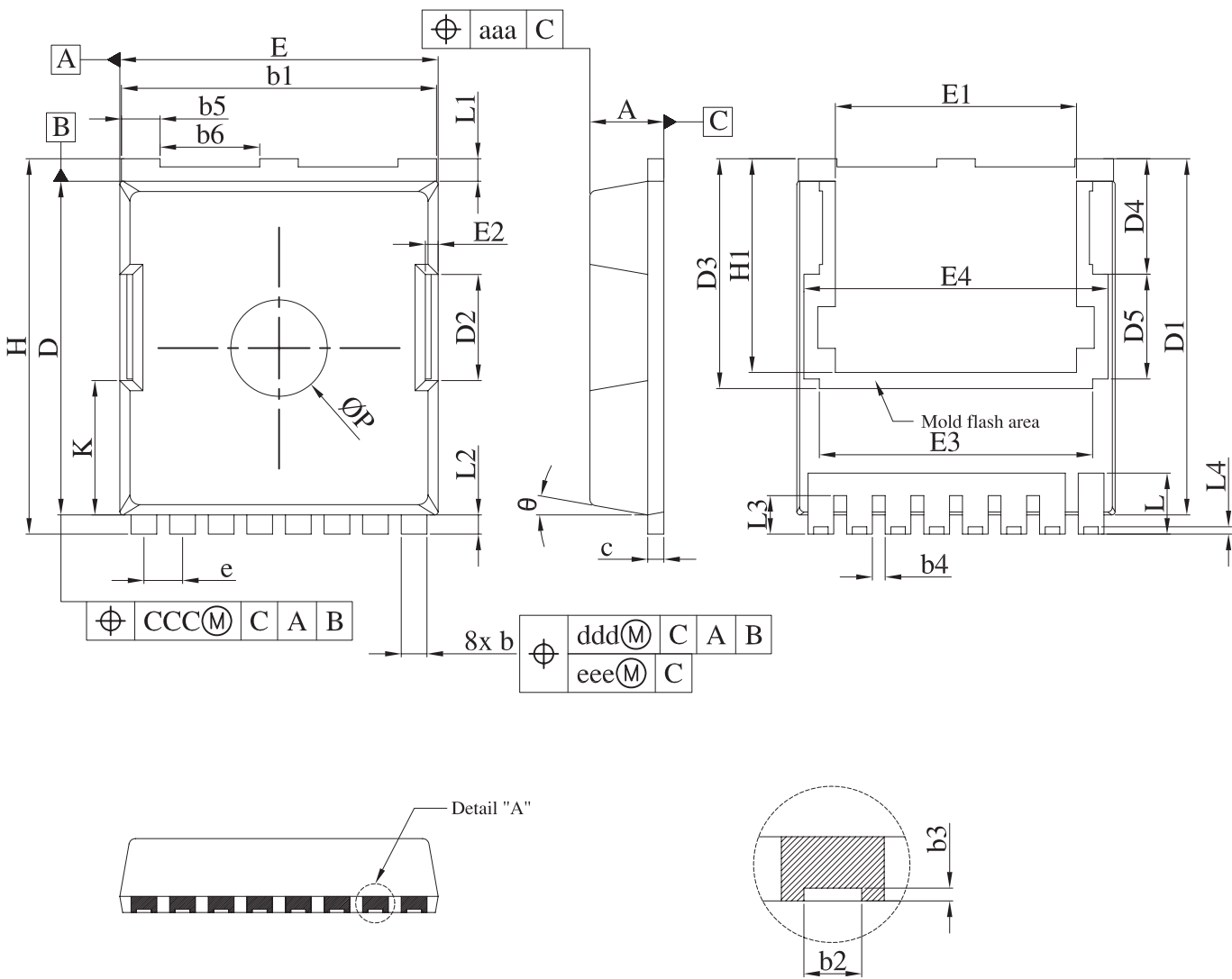
TOLL-8 Unit :mm
