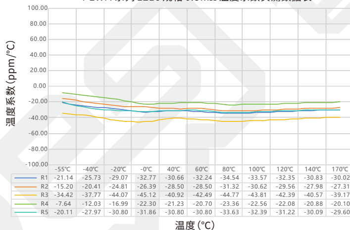
PEWM 系列 1216 规格 0.5mΩ 温度系数实测数据表
