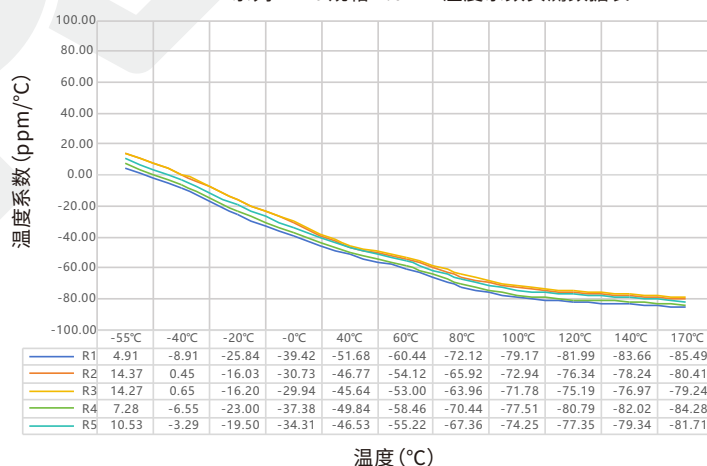
PEWM 系列 1216 规格 1.0mΩ 温度系数实测数据表
