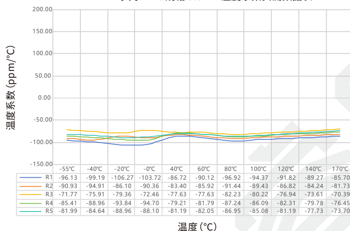
PEWM 系列 1216 规格 0.3mΩ 温度系数实测数据表
