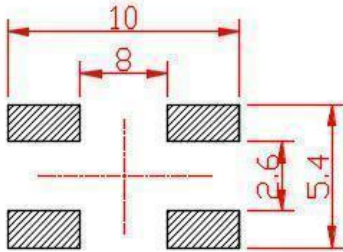
PCB. 焊接图
