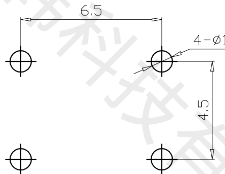
P.C.B焊接图
