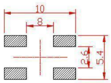
PCB. 焊接图
