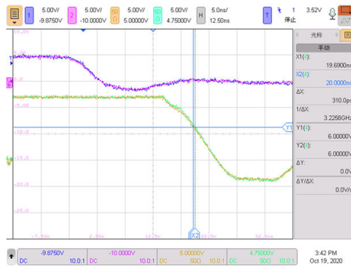
Figure 21. Falling Edge
