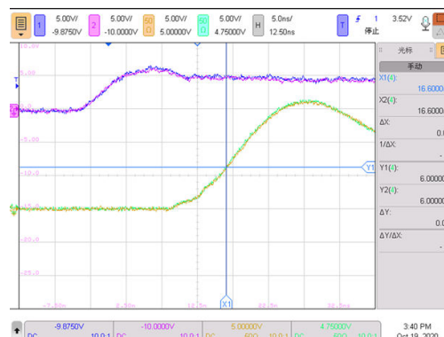
Figure 20. Rising Edge
