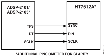
Figure 28. HT7512A to ADSP-2101/ADSP-2103 Interface
