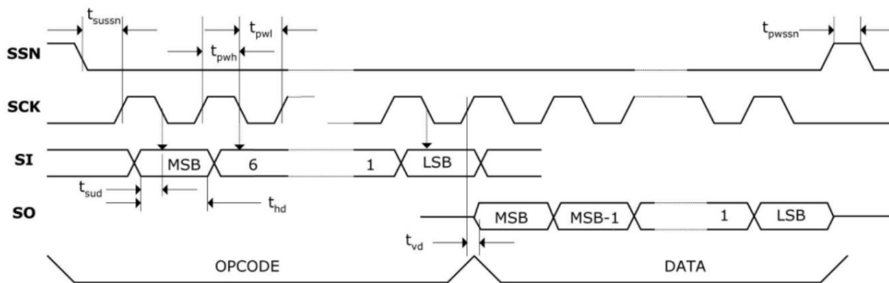
图 2. SPI 读时序
