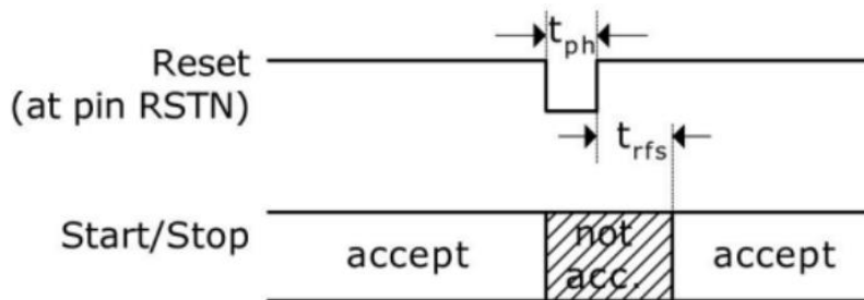
图 4. 系统复位时序
