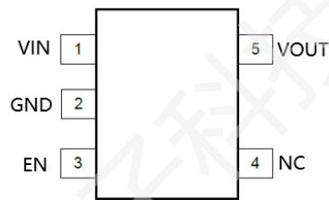
SOT23-5A
