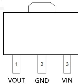
SOT89-3B
