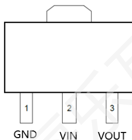
SOT89-3A
