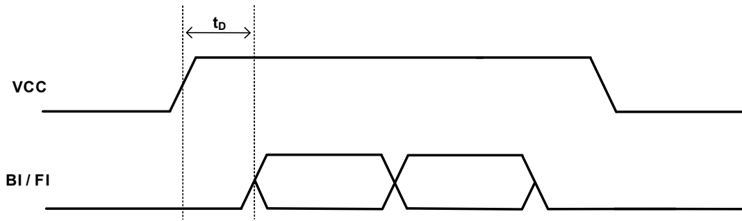
图 5. 上电时序图
