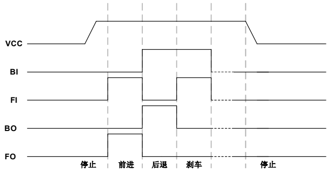
图 3. 输出时序图
